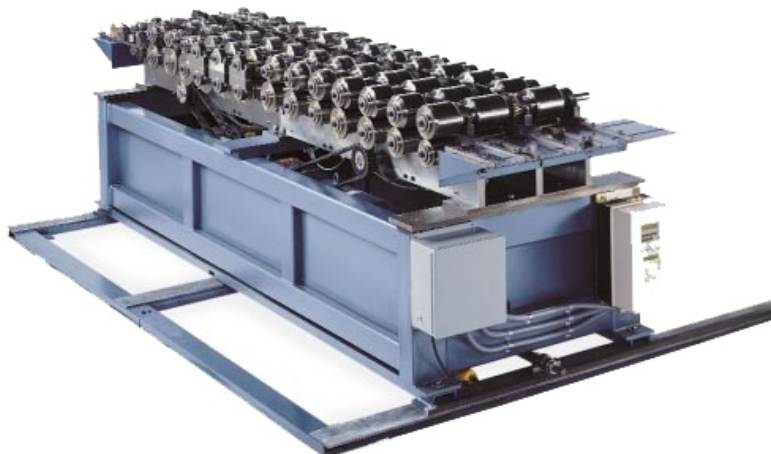
L-612 Trilex
