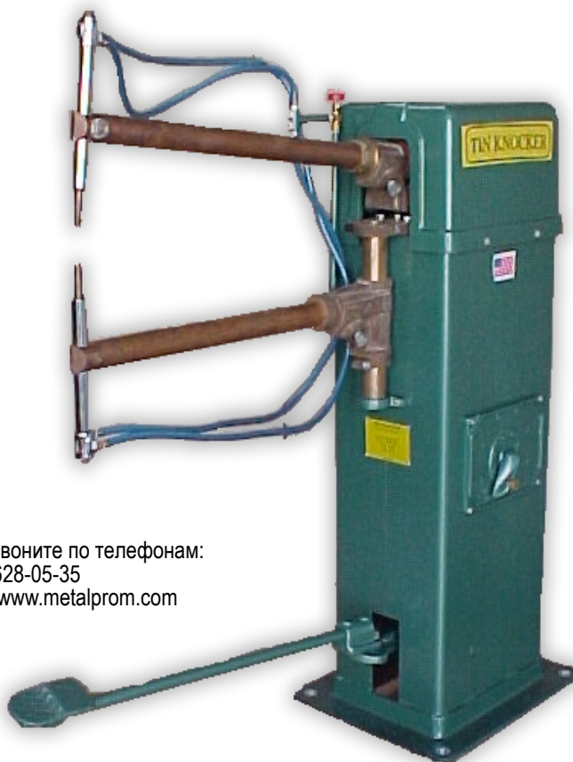
Станок для точечной сварки Spot Welder 1524
